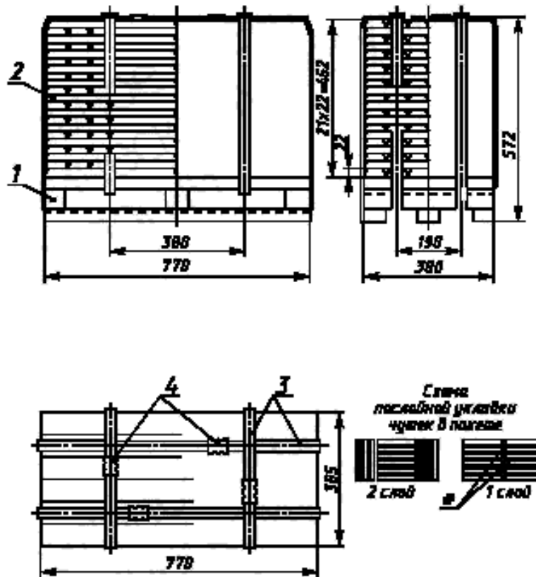
Схема укладки и крепления чушек кадмия в пакеты
