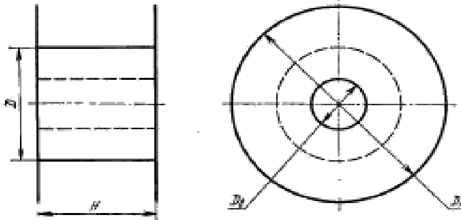
Размеры катушек для алюминиевой проволоки
