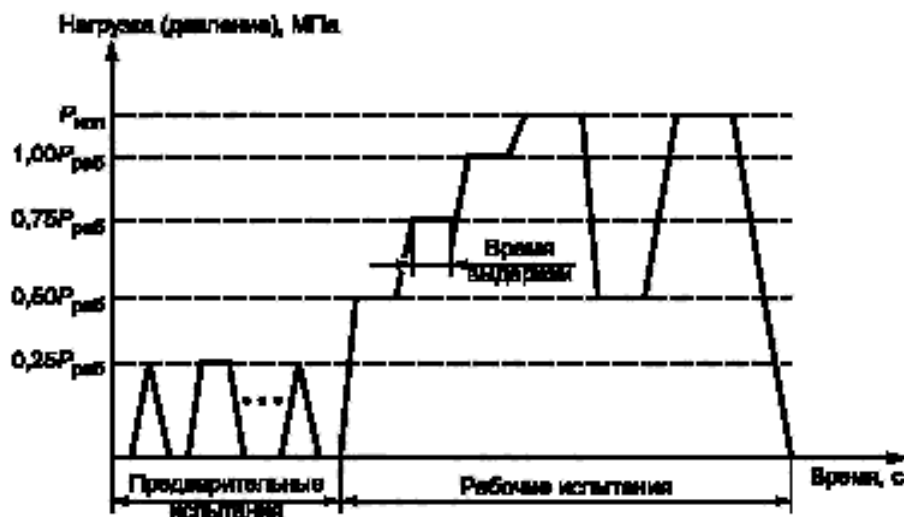
Рисунок 1 — Типовой график нагружения
