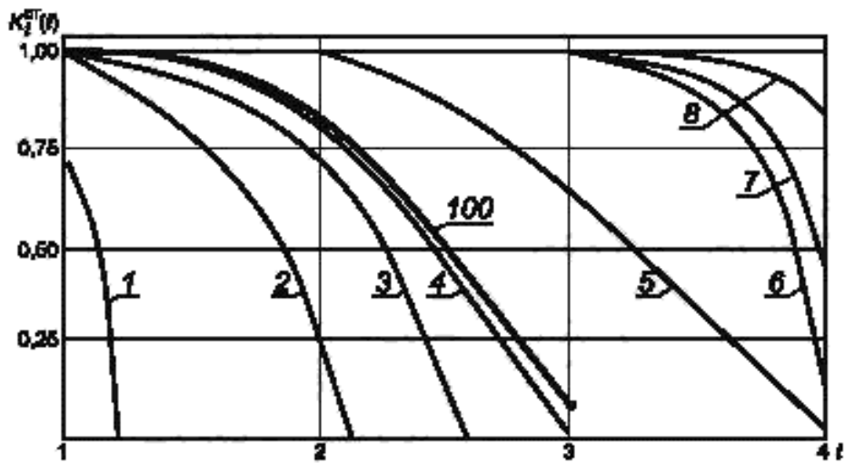
Рисунок А.2 — Кривая зависимости K_f(t) , нанесенная на серию тарировочных кривых
