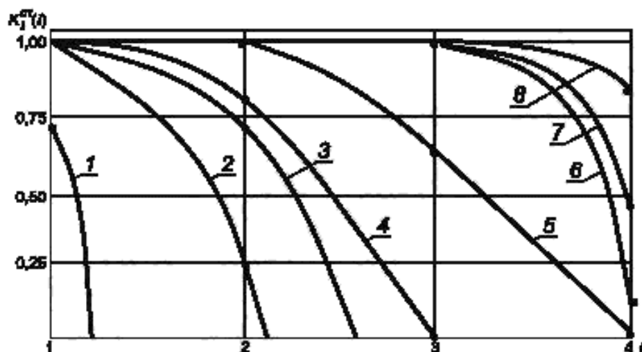
Рисунок А.1 — Серия тарировочных кривых K_i^{CT}(f)
