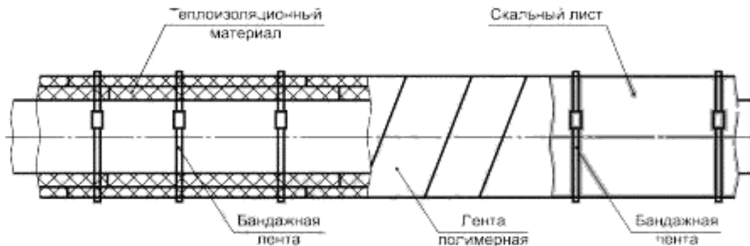
Рисунок 6.7 — Конструкция трубы в теплоизоляции с использованием скорлуп
