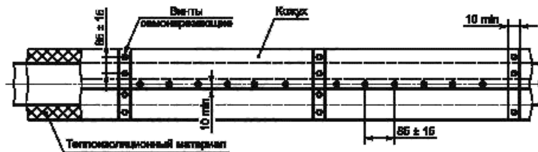
Рисунок 6.5 — Конструкция трубы в теплоизоляции
