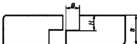
B — ширина паза, H — высота паза, S — толщина скорлупы
