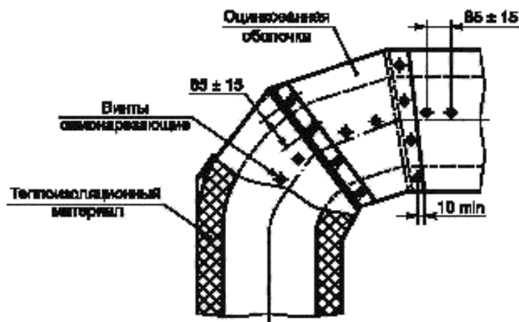
Рисунок 6.6 — Конструкция СДТ в теплоизоляции
