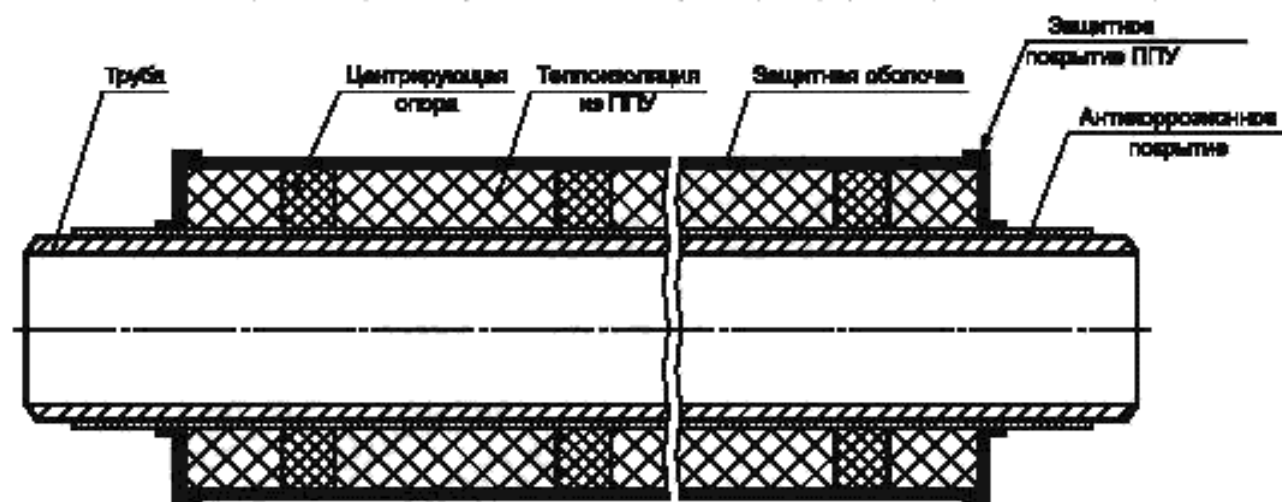
Рисунок 6.1 — Конструкция трубы в теплоизоляции
